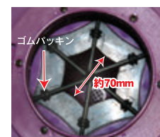
【挿入部：断面図】
