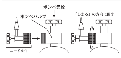
①矢印の方向へ回し、しっかりと手で閉め込んで下さい。 ※板レンチを使用しなくても、しっかりと閉まります。
